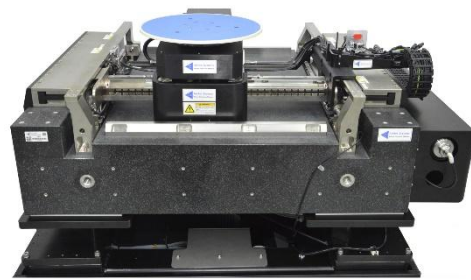
Linearservomotor und Linearführung von Akribis
